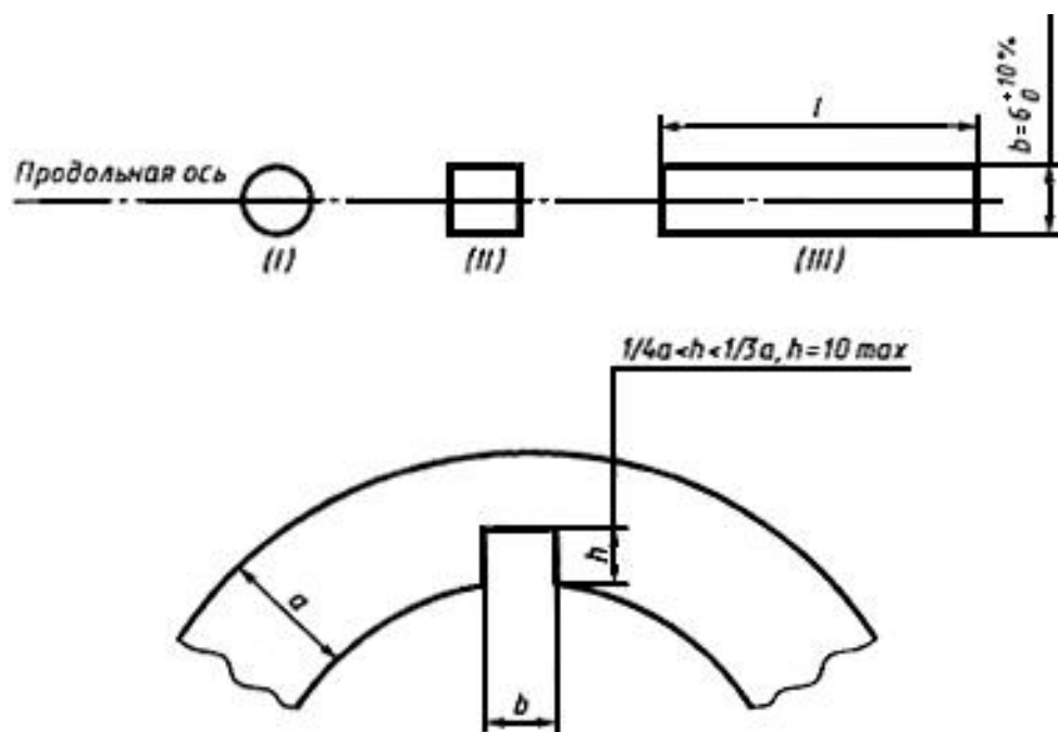
Рисунок 1 - Формы эталонных отверстия и выемок
